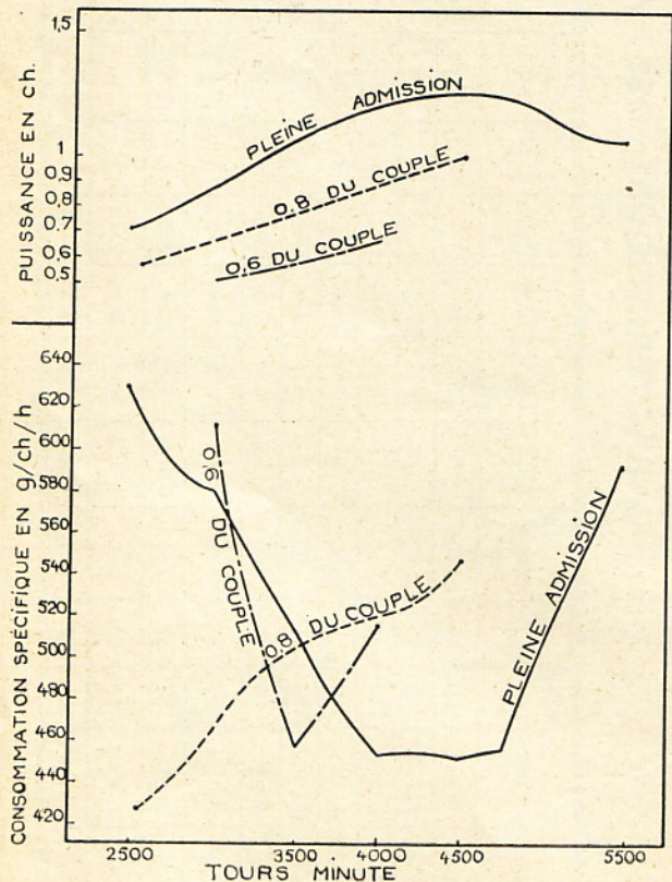
Courbes de consommation et de puissance
