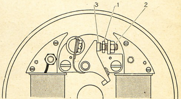
Réglage du rupteur du volant magnétique
