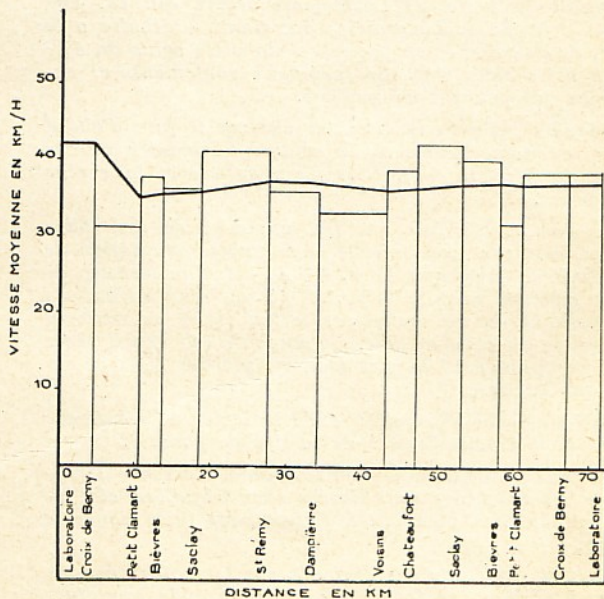
Courbe des vitesses
