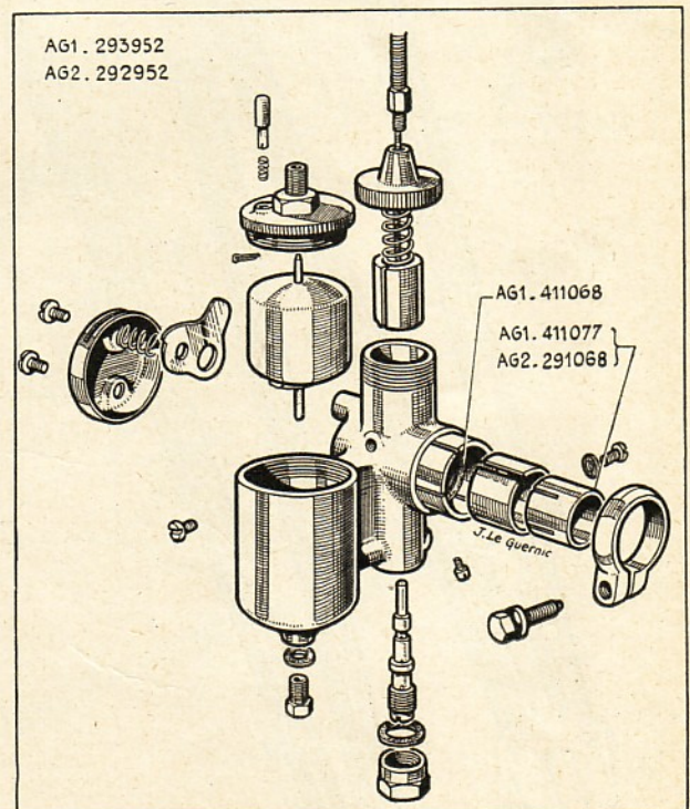
Vue du carburateur
